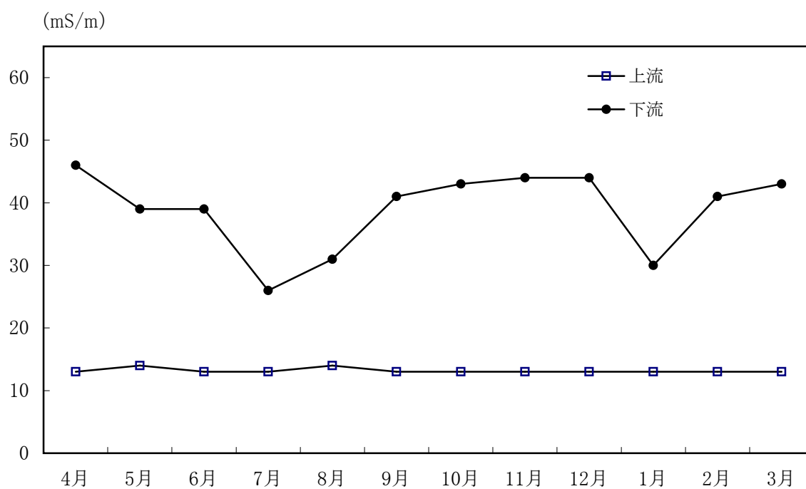
図－2 電気伝導率の経月変化
