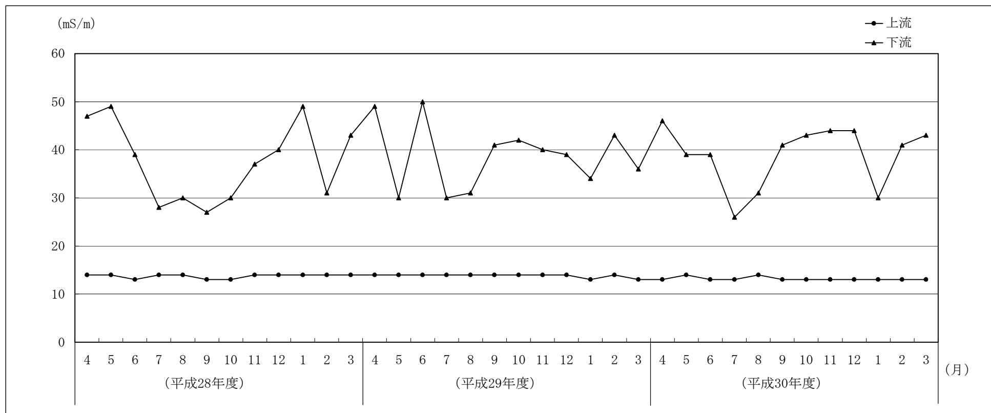
図－3 電気伝導率の推移
